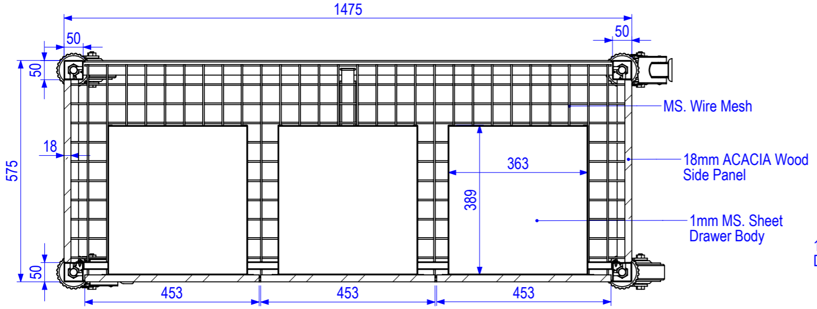
SECTION A-A
